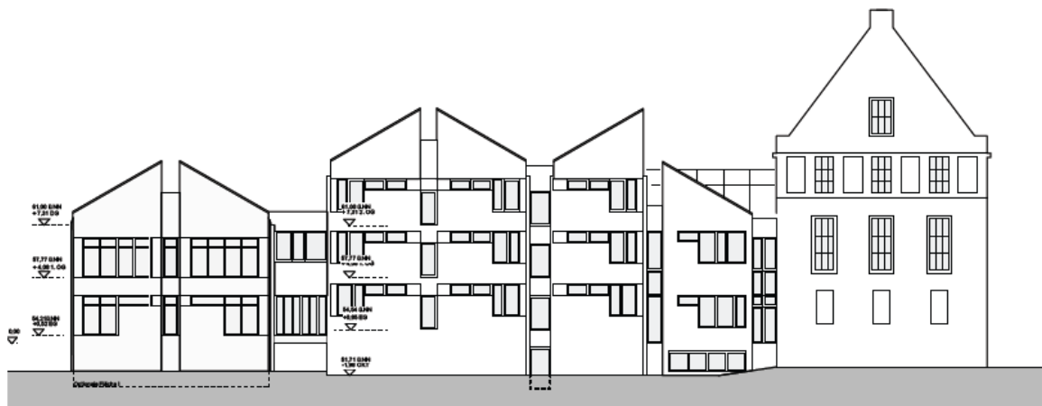
Ostansicht
